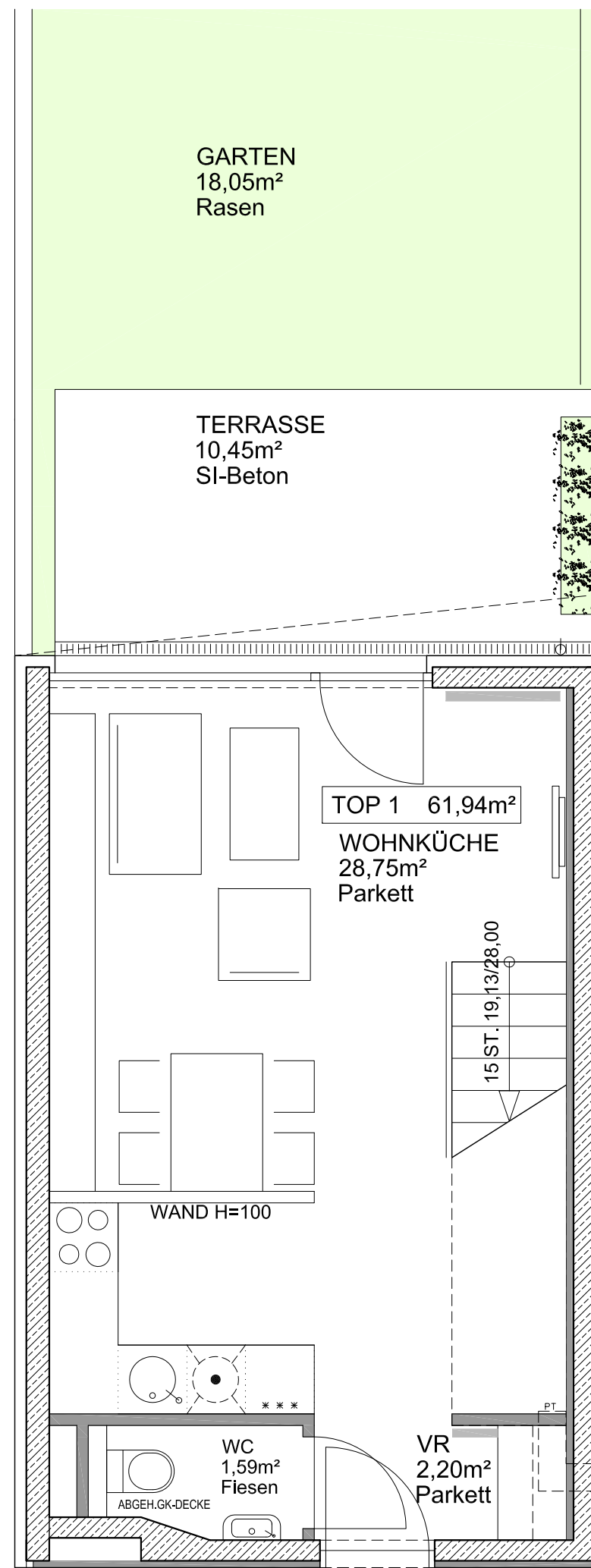
ERDGESCHOSS
